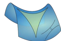
Geometría hiperbólica
